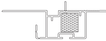
WF38036 80 mm cavity — jamb
